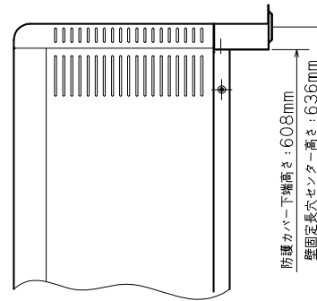
防護カバーが上下逆の場合
